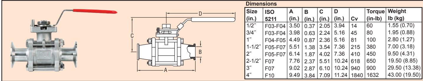
Dimensions
